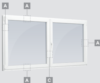
Dviejų varčių langas su judančiu statramsčiu
