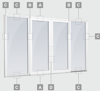
Ketverių dalių atverčiamos-stumdomos durys. Stumdomos varčios viduryje
